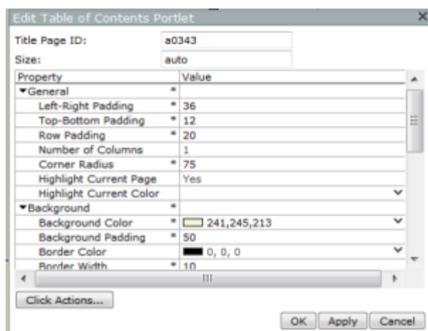
Figure 1 - La boîte de dialogue Édition du Table Of Contents Portlet
